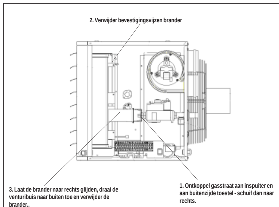
Figuur 14 - Werkwijze om brander te verwijderen
