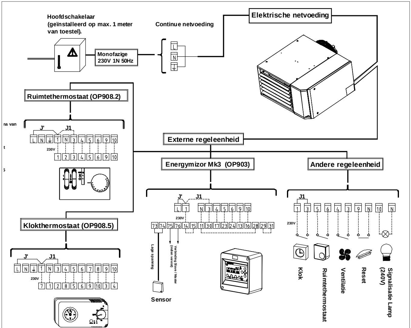
Figuur 9 : Aansluitingen op klemmenbord
