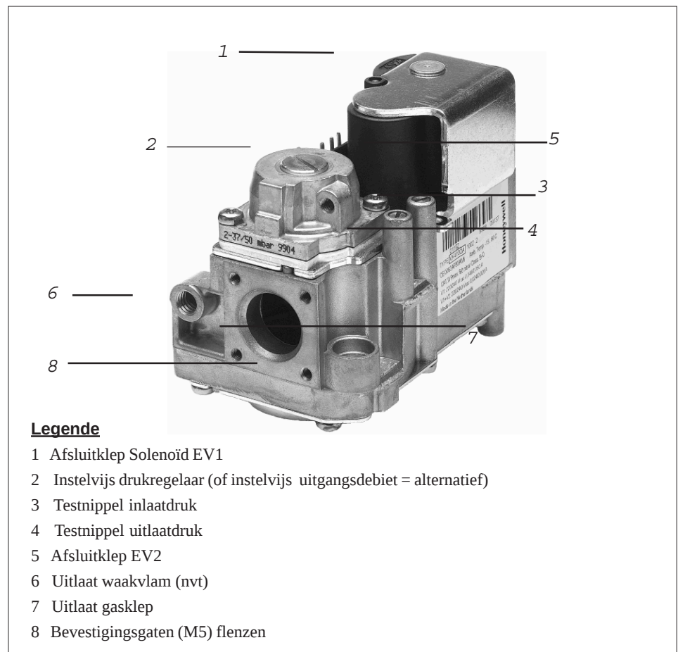
Figuur 10a : HONEYWELL Gasklep (types 008-2 -> 030-2)
